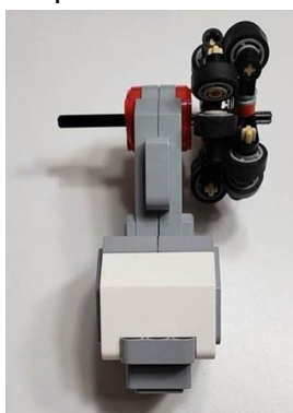
Ejemplo de rueda omnidireccional legal
